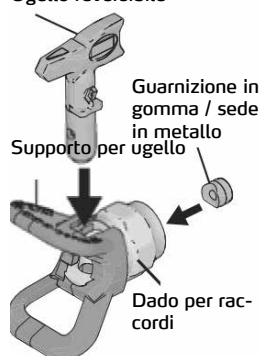
Ugello reversibile
